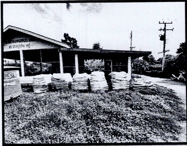
ภาพการจัดหาวัสดุ (ยางมะตอยสำเร็จรูป) และการดำเนินงานซ่อมแซมถนนสายสัมพันธ์ ๒ หมู่ที่ ๓ บ้านเชิงศิรี เมื่อวันที่ ๒ - ๓ กันยายน ๒๕๖๕
