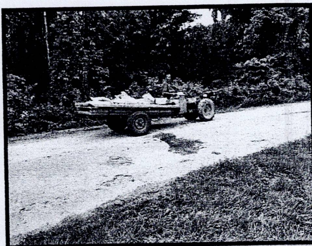
ภาพการจัดหาวัสดุ (ยางมะตอยสำเร็จรูป) และการดำเนินงานซ่อมแซมถนนสายสัมพันธ์ ๒ หมู่ที่ ๓ บ้านเชิงคีรี เมื่อวันที่ ๒ - ๓ กันยายน ๒๕๖๕
